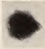
Strain TA.
